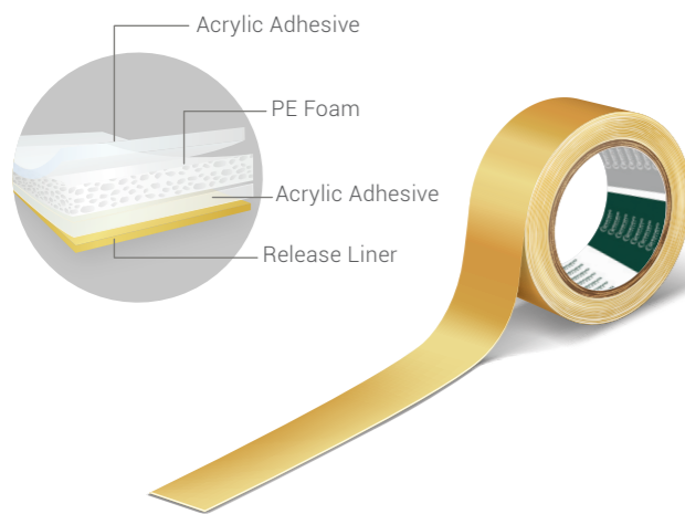
PE/PU Foam Double Sided PE Foam Tape
